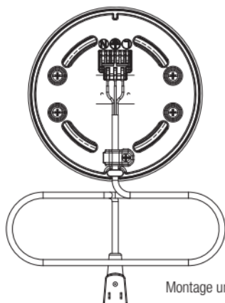
Gabarit de montage universel
